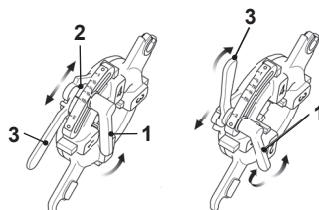
STANDARD - DIE HEAD
