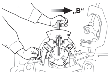
AUTOMATIC - DIE HEAD
