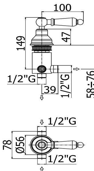
DISEGNO TECNICO
